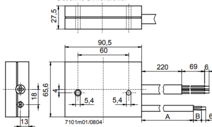
Desenho Dimensional
